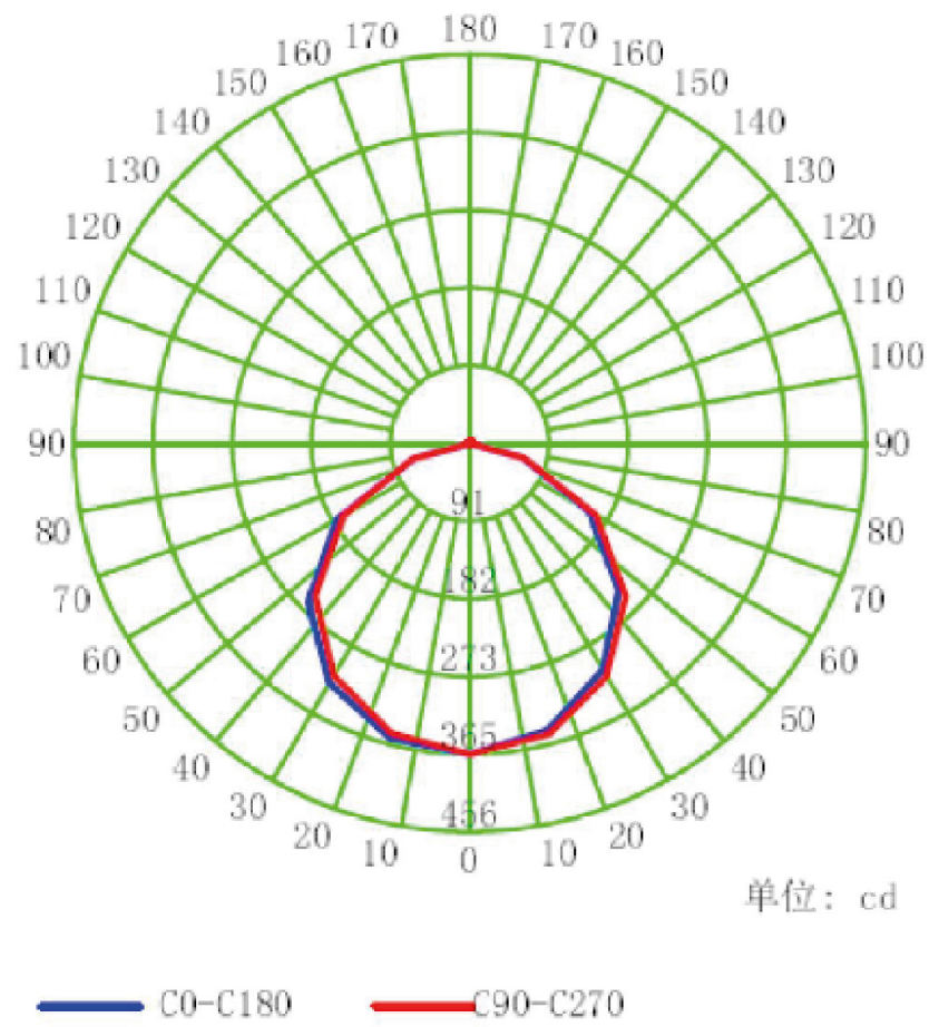
配光曲线
