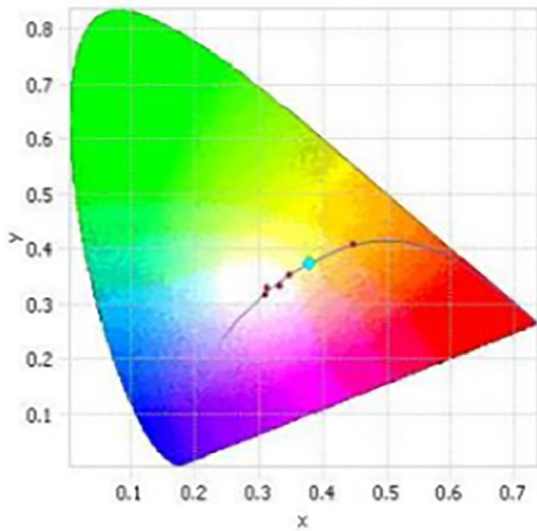
CIE 1931, 2 Degree
