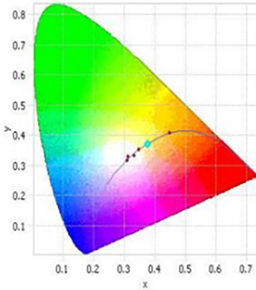
CIE 1931, 2 Degree
