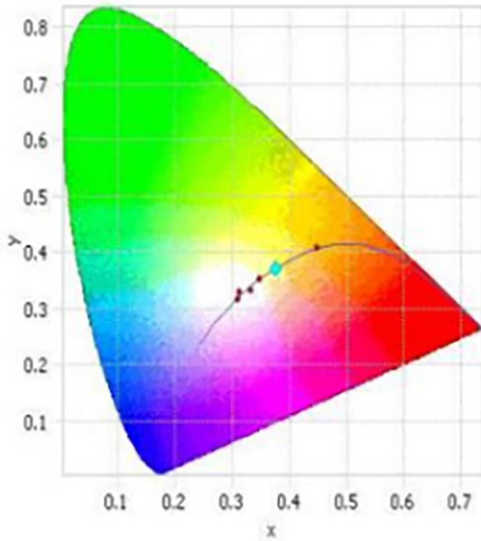
CIE 1931, 2 Degree
