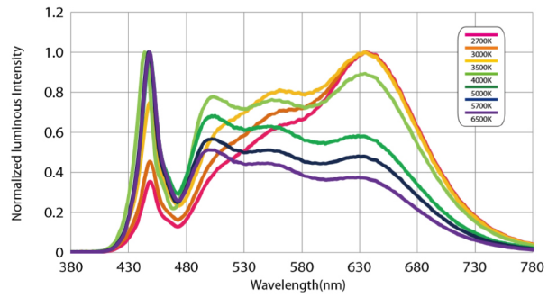
Color Spectrum ( T_c=25^{\circ}\text{C} , I_f=450\text{mA} )
