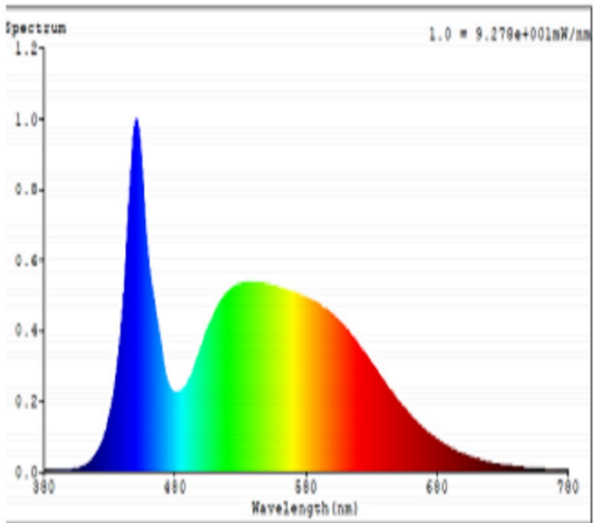
IK03-30W 6500K_Light source
