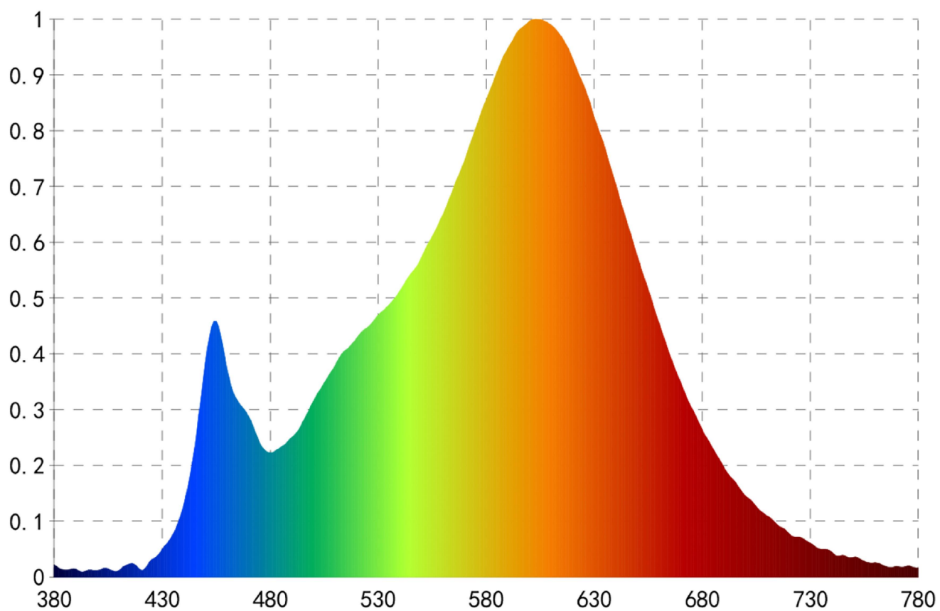
相对光谱
